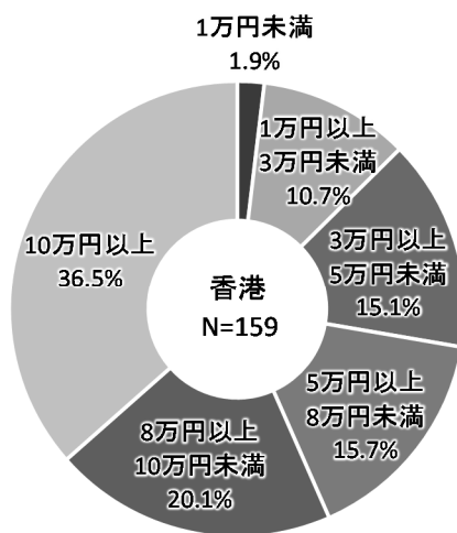
図 全体（香港）
