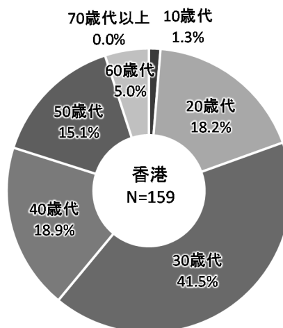
図 年齢（香港）
