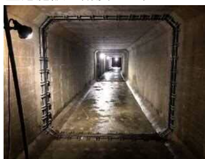
【 幹線排水路の耐震対策工事 (県営名古屋空港) 】
