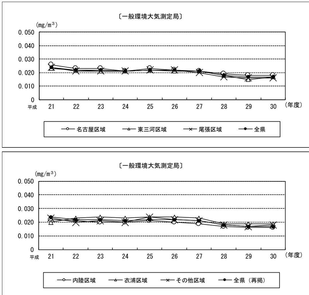
図1-6 一般環境大気測定局における浮遊粒子状物質の区域別年平均値の経年変化
