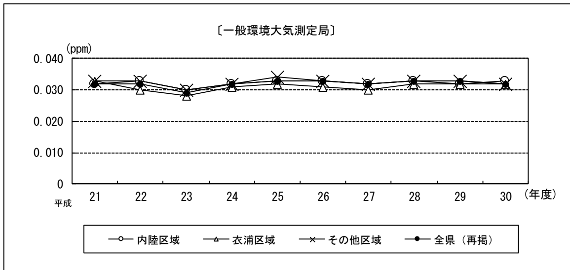
図1-7 一般環境大気測定局における光化学オキシダントの区域別年平均値の経年変化
