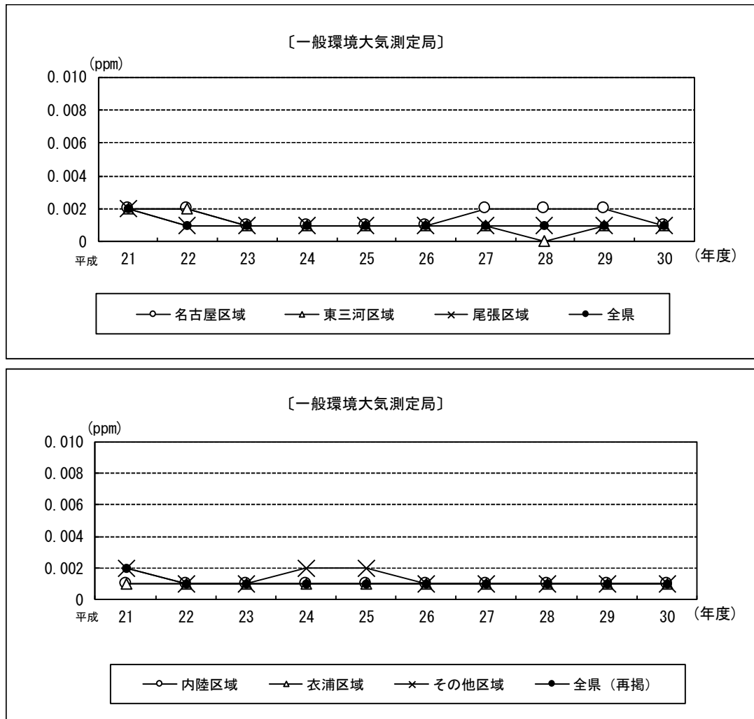
図1-3 一般環境大気測定局における二酸化硫黄の区域別年平均値の経年変化
