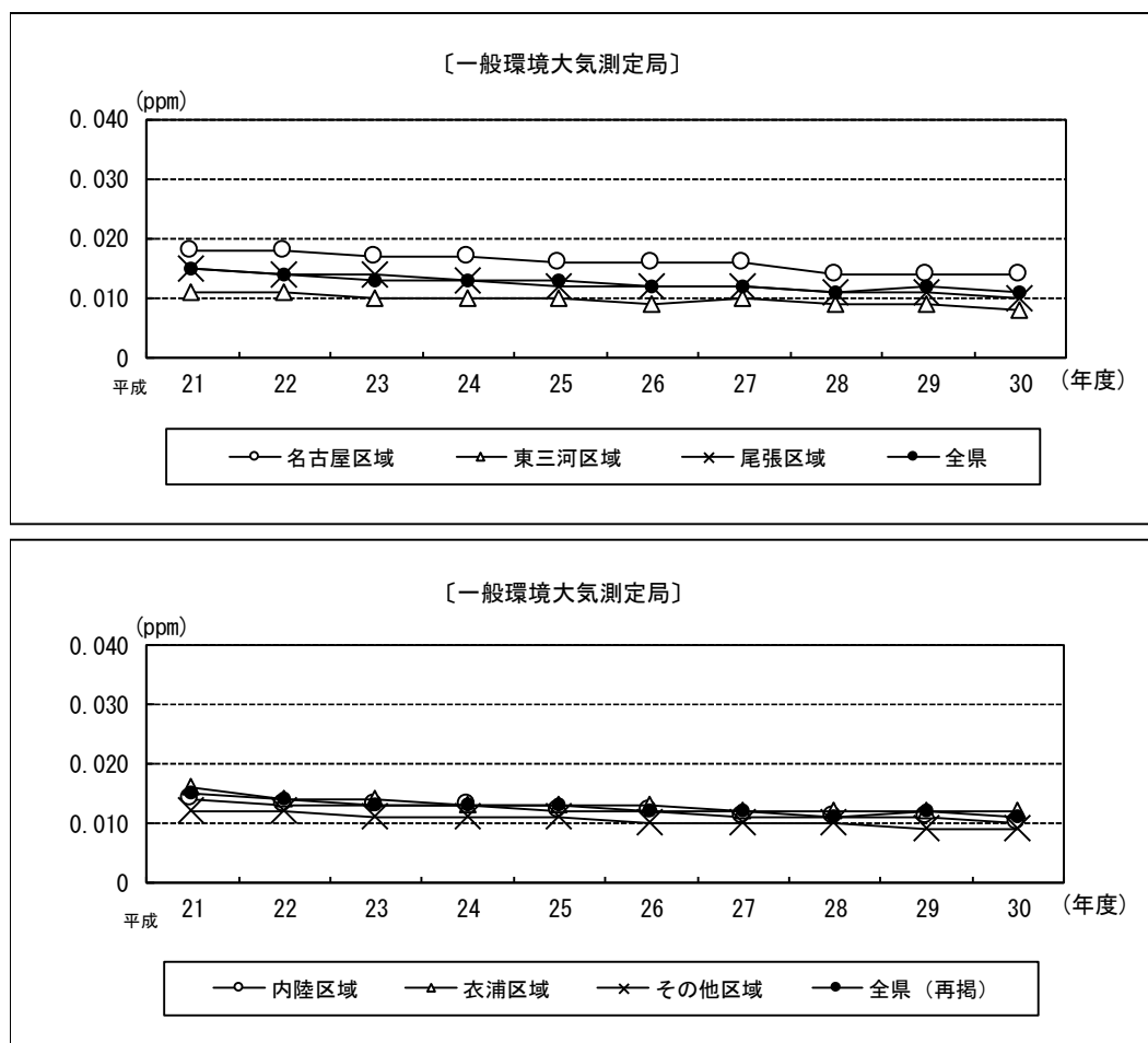
図1-4 一般環境大気測定局における二酸化窒素の区域別年平均値の経年変化
