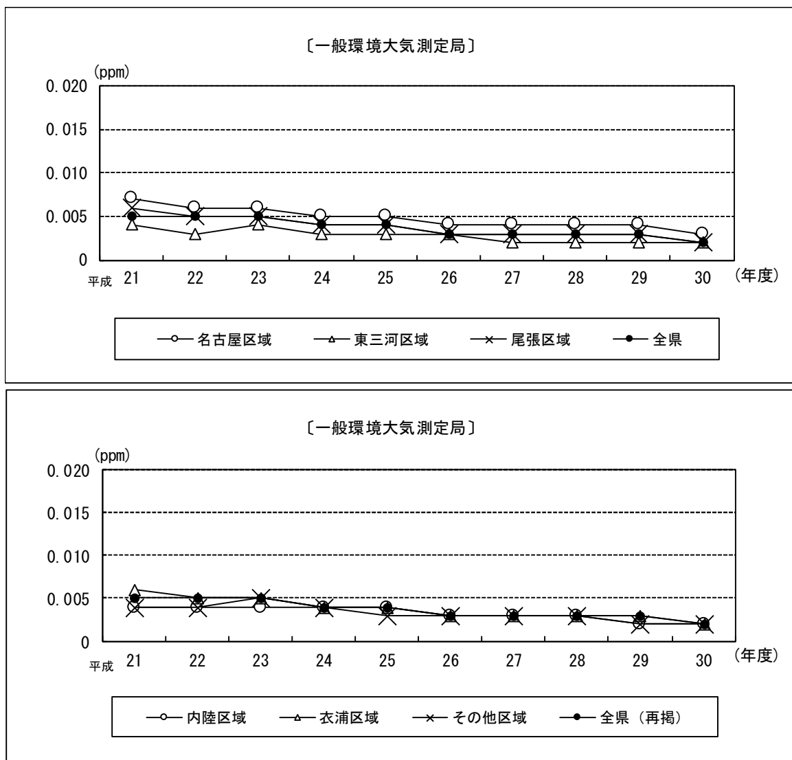
図1-5 一般環境大気測定局における一酸化窒素の区域別年平均値の経年変化
